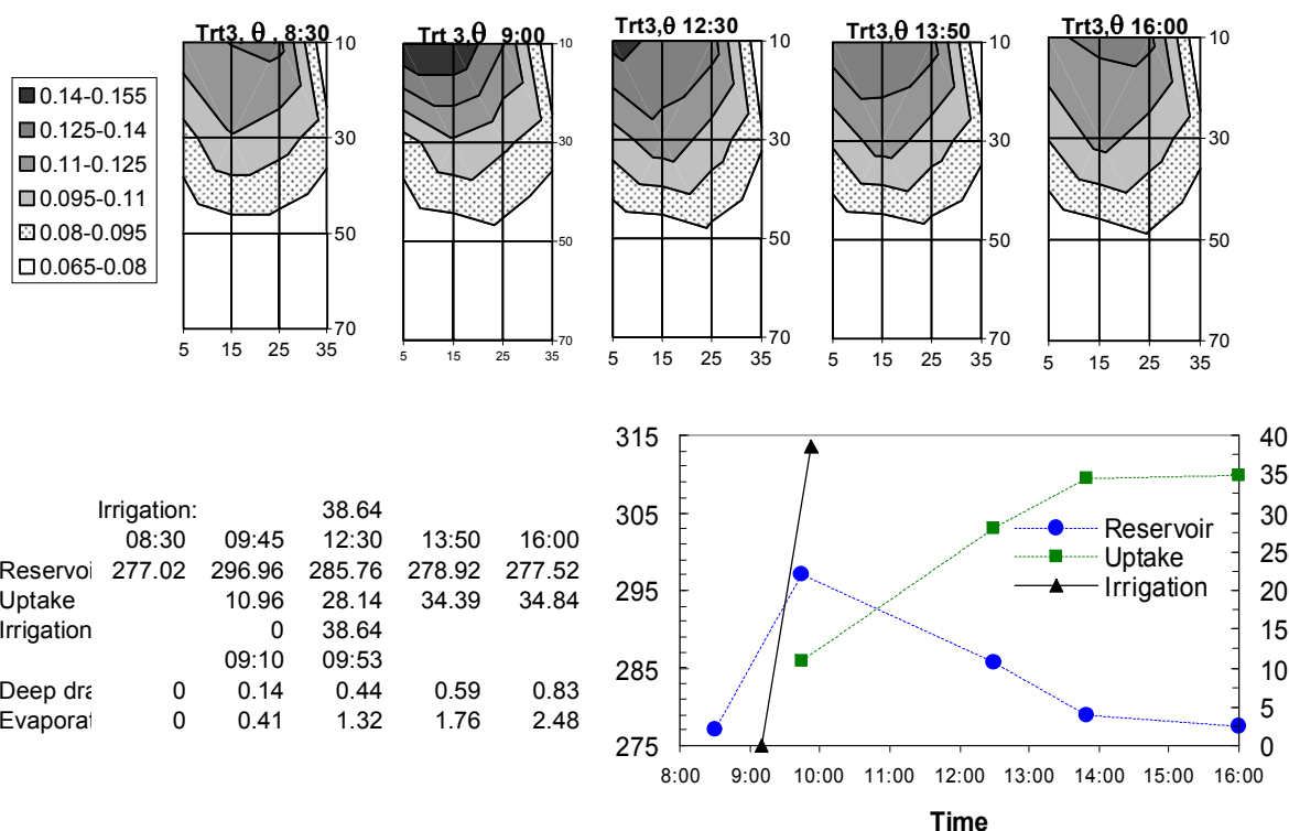
איור 6. למעלה: מהלך יומי של תכולת הרטיבות בטיפול 3, השקיה גבוהה שלוחה אחת (24 ביולי). למטה: מאזן מים מקורב עם אמדן זהיר להתאדות מפני השטח ולדליפה לעומק הקרקע.
