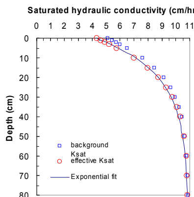
איור 4. הערכה לפחיתת המוליכות ההידראולית ברוויה בחתך הקרקע כתוצאה מנוכחות שורשים.
